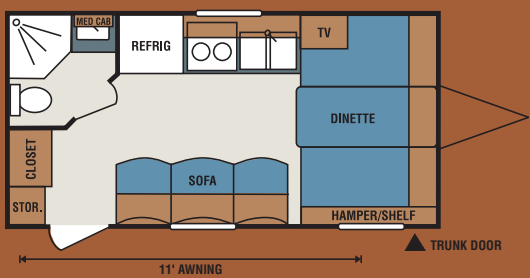
CL162 • UVW 2930 • Dry Hitch Wt. 320 • NCC 570 • Length 20' 5"
