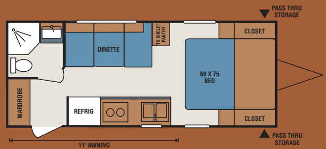
CL180 • UVW 3580 • Dry Hitch Wt. 320 • NCC 920 • Length 23' 8"
