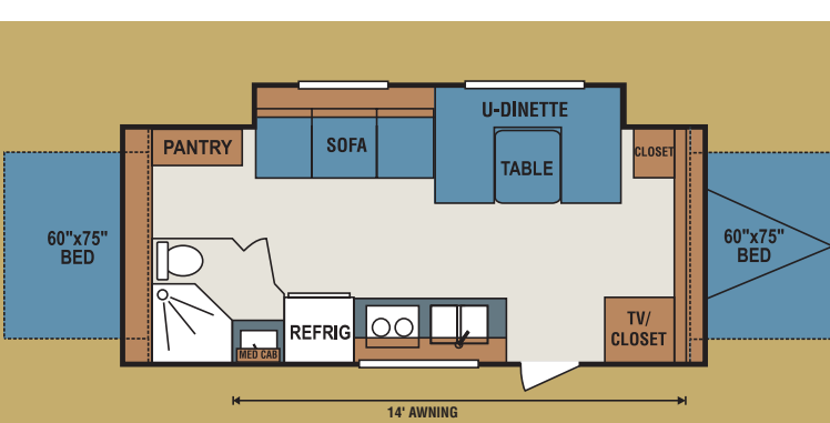
22CP • UVW 4340 • Dry Hitch Wt. 550 • NCC 1160 • Length 23' 8"
