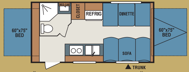
20C • UVW 3340 • Dry Hitch Wt. 400 • NCC 1160 • Length 20' 8"
