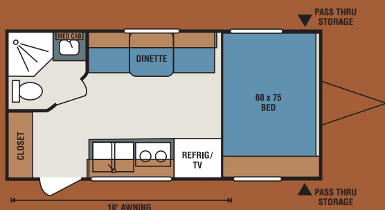
CL164 • UVW 2820 • Dry Hitch Wt. 290 • NCC 680 • Length 20' 5"
