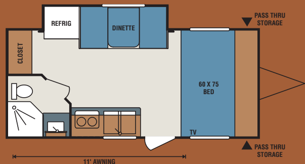
CL163 • UVW 3010 • Dry Hitch Wt. 330 • NCC 490 • Length 20' 5"
