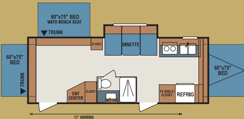
23CR • UVW 4490 • Dry Hitch Wt. 740 • NCC 1510 • Length 26' 3"
