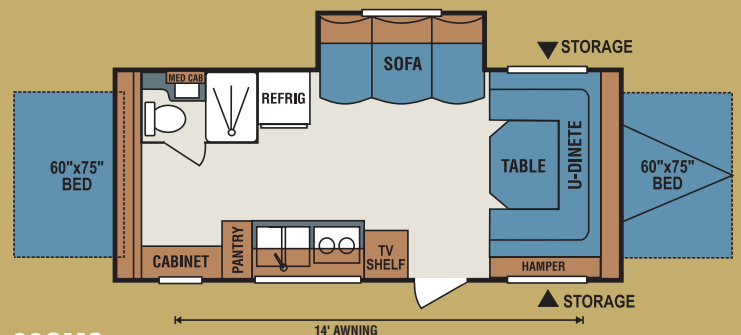
23CMS • UVW 4090 • Dry Hitch Wt. 460 • NCC 1410 • Length 24' 7"
