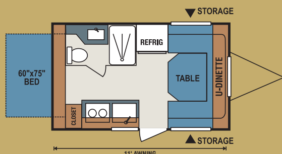
16C • UVW 2780 • Dry Hitch Wt. 290 • NCC 720 • Length 17' 9"
