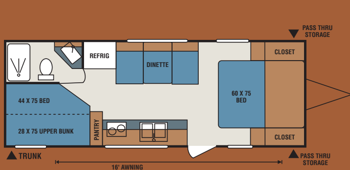
CL230 • UVW 4020 • Dry Hitch Wt. 490 • NCC 1480 • Length 27'
