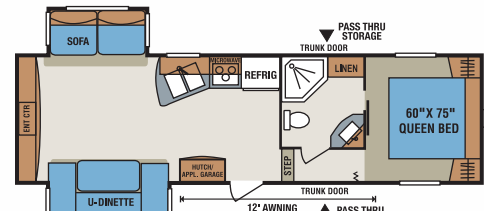
S265RE • UVW 7673 • Dry Hitch Wt. 1590 • NCC 2327 • Length 30'9"
