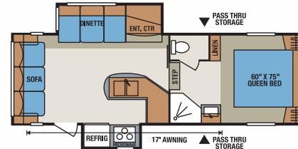
S245RL2 • UVW 7270 • Dry Hitch Wt. 1337 • NCC 2530 • Length 27'6"
