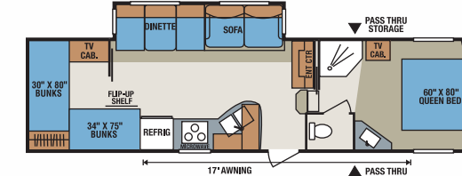
S315BH • UVW 8376 • Dry Hitch Wt. 1734 • NCC 2924 • Length 34'
