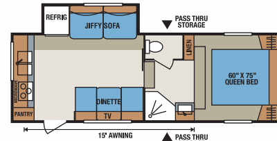
S235RK • UVW 6007 • Dry Hitch Wt. 974 • NCC 1893 • Length 25'3"
