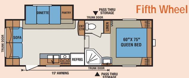
S237LE • UVW 6147 • Dry Hitch Wt. 1397 • NCC 1853 • Length 27'
