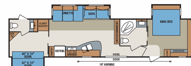
S391FL2 • UVW 8797 • Dry Hitch Wt. 1381 • NCC 2703 • Length 41'5"
