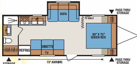
S251RB • UVW 4960 • Dry Hitch Wt. 513 • NCC 1340 • Length 26'
