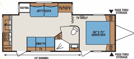
S261RK • UVW 5164 • Dry Hitch Wt. 563 • NCC 1836 • Length 28'9"
