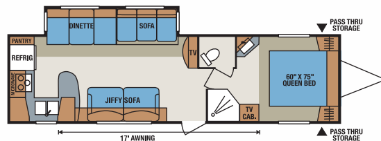
S310RKS • UVW 6806 • Dry Hitch Wt. 649 • NCC 3194 • Length 33'9"
