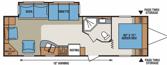
S290RE • UVW 6437 • Dry Hitch Wt. 666 • NCC 3563 • Length 32'10"
