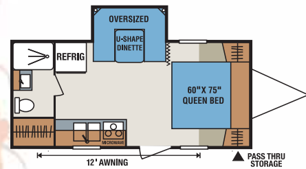
S202SLE • UVW 3844 • Dry Hitch Wt. 450 • NCC 2156 • Length 22'5"
