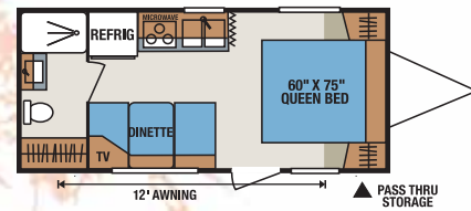
S202LE • UVW 3458 • Dry Hitch Wt. 415 • NCC 2542 • Length 21'11"
