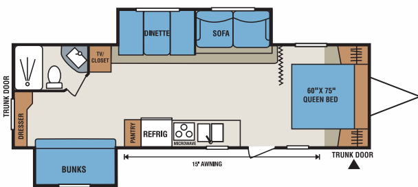
S318LE • UVW 5540 • Dry Hitch Wt. 547 • NCC 1460 • Length 31'11"
