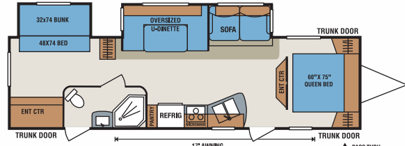
S321BH • UVW 7309 • Dry Hitch Wt. 734 • NCC 2691 • Length 34'3"
