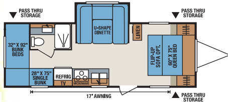
S240BHS • UVW 4526 • Dry Hitch Wt. 582 • NCC 1954 • Length 27'4"
