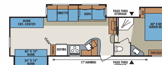
S325BH3 • UVW 9217 • Dry Hitch Wt. 1967 • NCC 2283 • Length 34'4"
