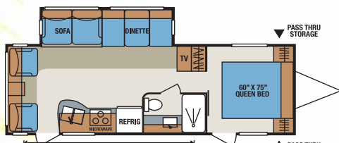
S280RL • UVW 6344 • Dry Hitch Wt. 682 • NCC 3656 • Length 30'
