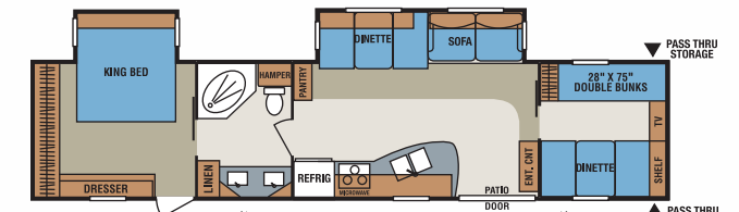
S383BH2 • UVW 9013 • Dry Hitch Wt. 1121 • NCC 2487 • Length 40'4"
