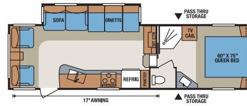
S285RL • UVW 7784 • Dry Hitch Wt. 1605 • NCC 3316 • Length 31'
