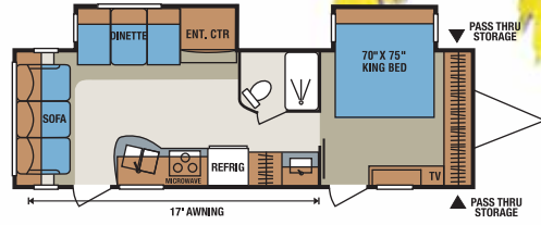
S290KB • UVW 6929 • Dry Hitch Wt. 1029 • NCC 3071 • Length 32'10"
