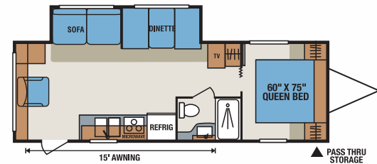
S280LE • UVW 4916 • Dry Hitch Wt. 617 • NCC 2084 • Length 29'10"
