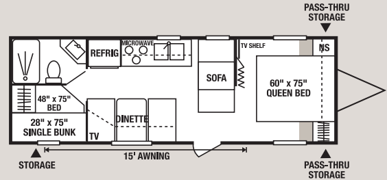
28JB • UVW 4830 • Dry Hitch Wt. 620 • NCC 2170 • Length 29'5"
