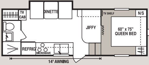
22JFS • UVW 5240 • Dry Hitch Wt. 1120 • NCC 1760 • Length 23'8"
