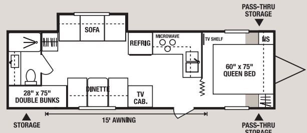
29JBS • UVW N/A • Dry Hitch Wt. N/A • NCC N/A • Length N/A
