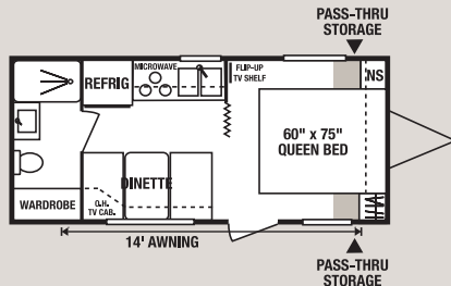
20J • UVW 3840 • Dry Hitch Wt. 510 • NCC 2160 • Length 21'8"
