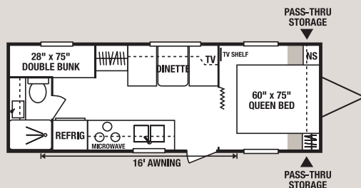
24JB • UVW 4300 • Dry Hitch Wt. 450 • NCC 2700 • Length 25'8"
