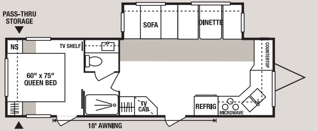
29JSS • UVW 6320 • Dry Hitch Wt. 1110 • NCC 3680 • Length 30'
