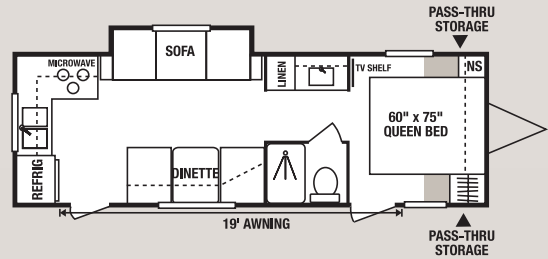
26JS • UVW 4870 • Dry Hitch Wt. 440 • NCC 2130 • Length 27'3"
