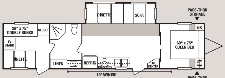
38JSS • UVW 7780 • Dry Hitch Wt. 700 • NCC 2220 • Length 38'8"
