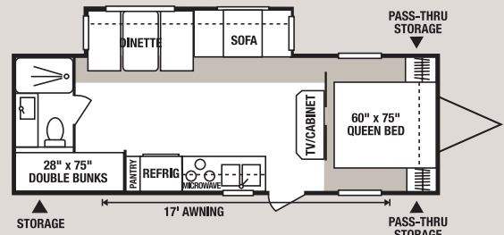
28JBSS • UVW 6130 • Dry Hitch Wt. 780 • NCC 3870 • Length 29'
