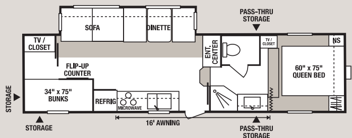
29JFSS • UVW 7350 • Dry Hitch Wt. 1340 • NCC 2650 • Length 29'
