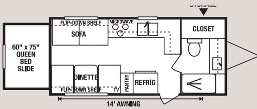
21JQ • UVW 4286 • Dry Hitch Wt. 510 • NCC 2714 • Length 22'4"
