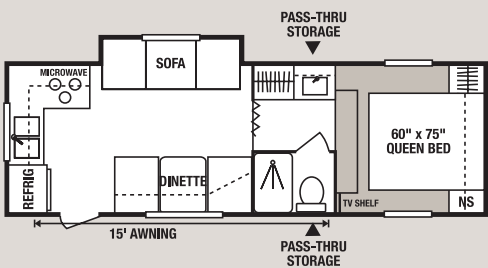
23JFS • UVW 5440 • Dry Hitch Wt. 830 • NCC 1560 • Length 23'8"
