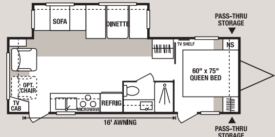
28JSS • UVW 6230 • Dry Hitch Wt. 660 • NCC 3770 • Length 29'3"
