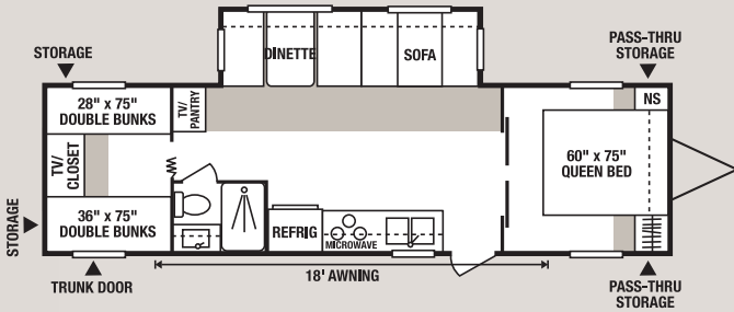
32JSS • UVW 6700 • Dry Hitch Wt. 660 • NCC 3940 • Length 33'6"
