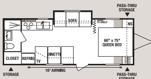
25JS • UVW 4590 • Dry Hitch Wt. 510 • NCC 2410 • Length 25'6"
