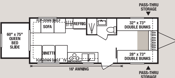
25JQ • UVW 4810 • Dry Hitch Wt. 460 • NCC 2190 • Length 24'9"
