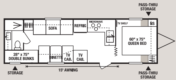
29JB • UVW 4800 • Dry Hitch Wt. 650 • NCC 2200 • Length 29'5"
