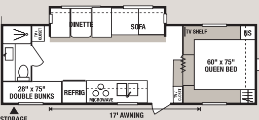
25JFS • UVW 6230 • Dry Hitch Wt. 1260 • NCC 3770 • Length 26'
