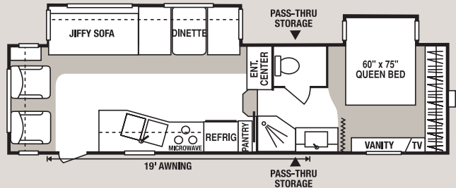
28JF2S • UVW 7390 • Dry Hitch Wt. 1600 • NCC 2610 • Length 29'8"
