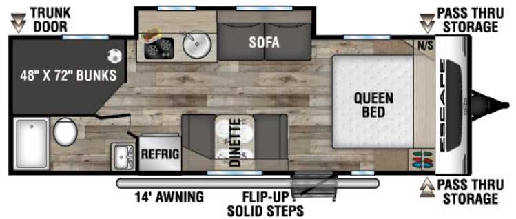
E231BH UYW - 4,140 | Exterior Length - 27' 3" | Sleeps - 8
