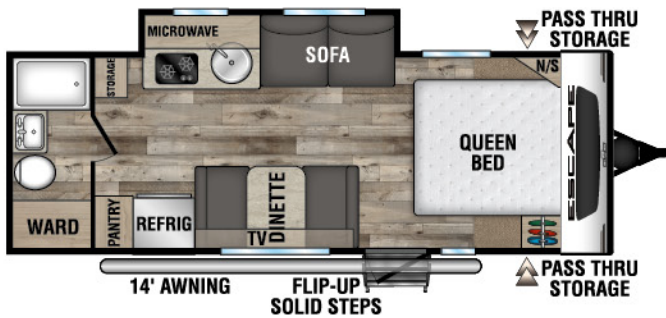
E211RB UYW - 3,840 | Exterior Length - 25' 2" | Sleeps - 4
