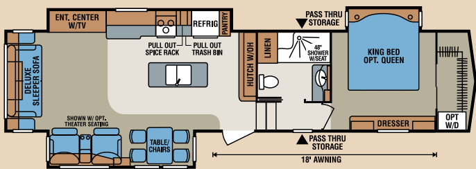
G370RLT UVW 11,686 • Dry Hitch Wt. 2,250 NCC 2,814 • Length 39' 6"
